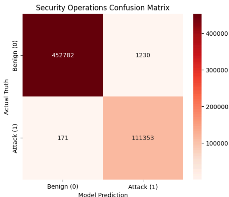
Σχήμα 5.1: Confusion Matrix των αποφάσεων των συμβάντων. Θεωρώντας ότι το σύνολο δοκιμής είναι μια προσομοίωση ημερήσιας δικτυακής κίνησης, το σύστημα κλήθηκε να λάβει αποφάσεις δρομολόγησης συμβάντων.
