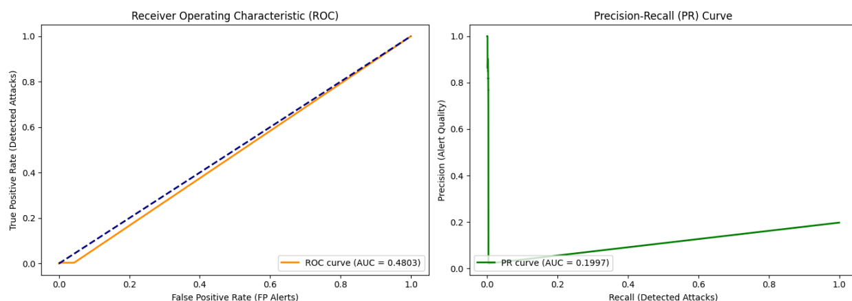
Σχήμα 5.2: Καμπύλες Λειτουργικού Χαρακτηριστικού Δέκτη (ROC) και Ακρίβειας-Ανάκλησης (Precision-Recall) για την αξιολόγηση των κατωφλίων.
