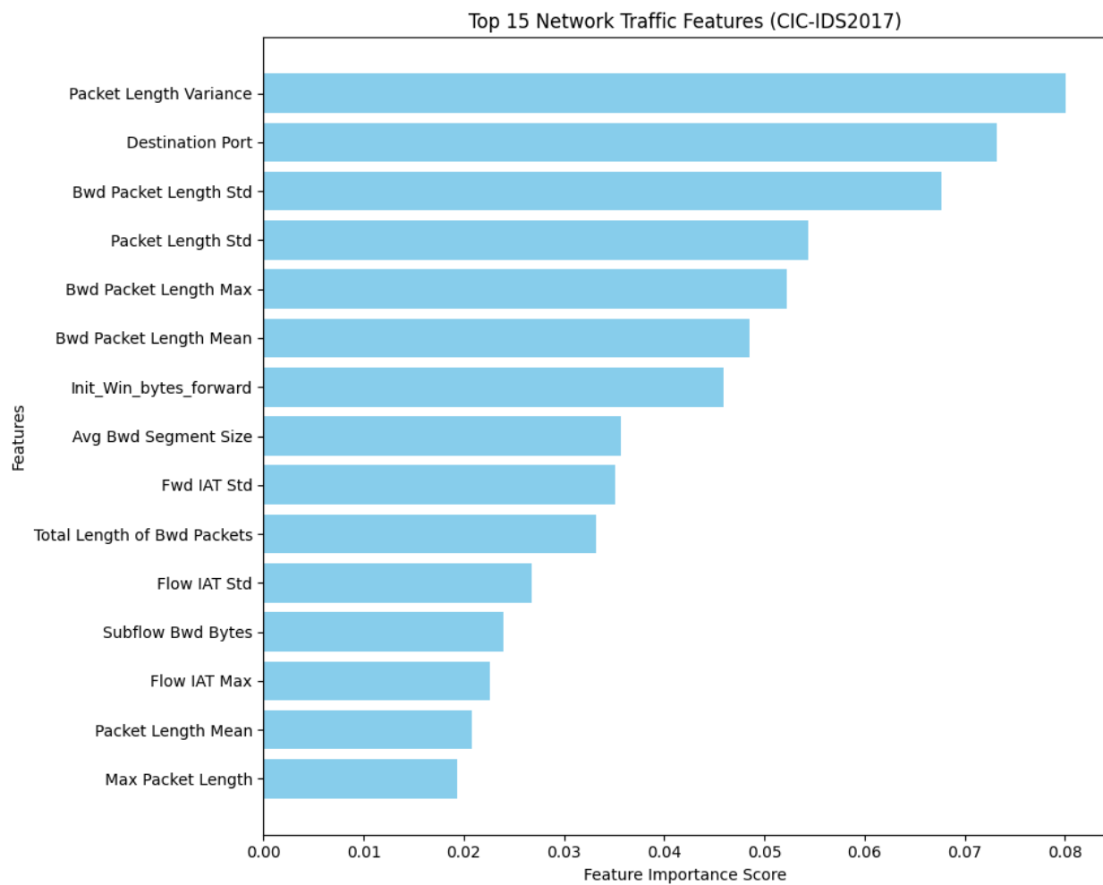
Σχήμα 3.1: Απεικόνιση των 15 σημαντικότερων δικτυακών μεταβλητών βάσει του κριτηρίου Gini Impurity του αλγορίθμου Random Forest.
