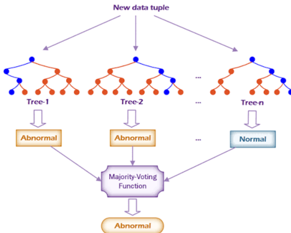
Σχήμα 4.1: Αρχιτεκτονική του αλγορίθμου Τυχαίου Δάσους (Random Forest) και ο μηχανισμός πλειοψηφικής ψηφοφορίας.
