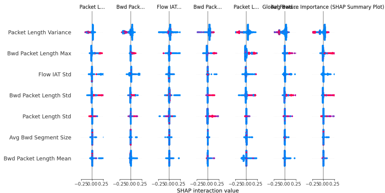
Σχήμα 5.3: Συνοπτικό γράφημα SHAP. Η θέση στον οριζόντιο άξονα δείχνει την επιρροή στο αποτέλεσμα (δεξιά αυξάνει την πιθανότητα "Επίθεσης"), ενώ το χρώμα (μπλε έως φούξια) υποδηλώνει την αρχική τιμή του χαρακτηριστικού.
