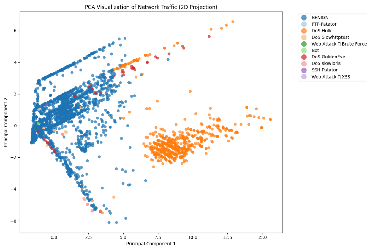
Σχήμα 3.2: Δισδιάστατη προβολή των δεδομένων μέσω PCA (Δείγμα 10.000 εγγραφών). Αναδεικνύεται η γεωμετρική απομάκρυνση των επιθέσεων όγκου, ενώ καταγράφεται ταξική επικάλυψη στις επιθέσεις εφαρμογών.
